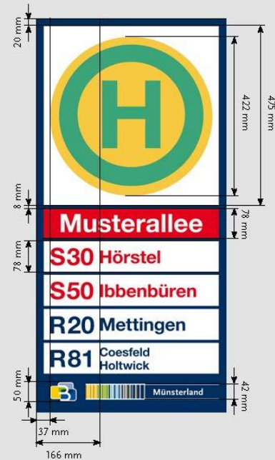
Vermaßung der Haltestellenfahne „WVG-Kompakt“
